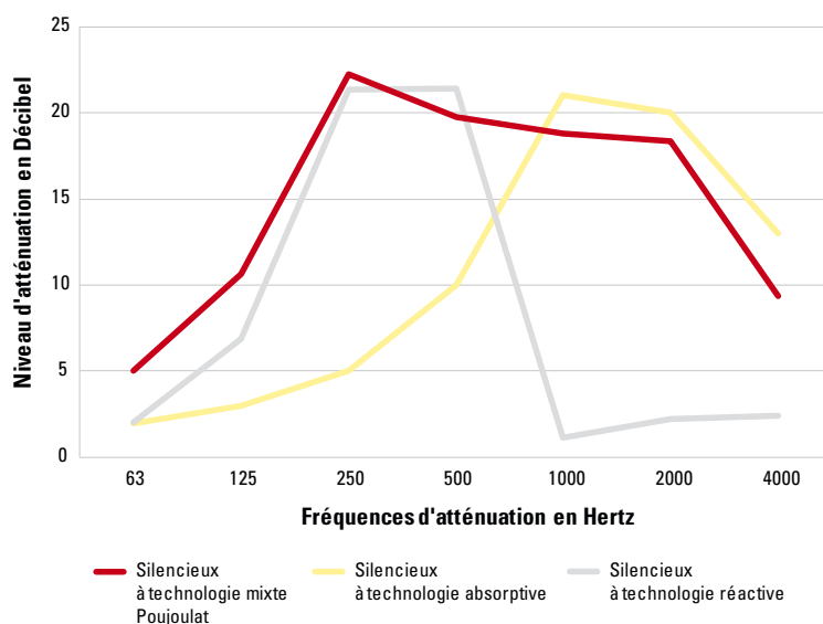
COURBES D'ATTÉNUATION SUIVANT DIFFÉRENTES TECHNOLOGIES POUR UN SILENCIEUX Ø 250
